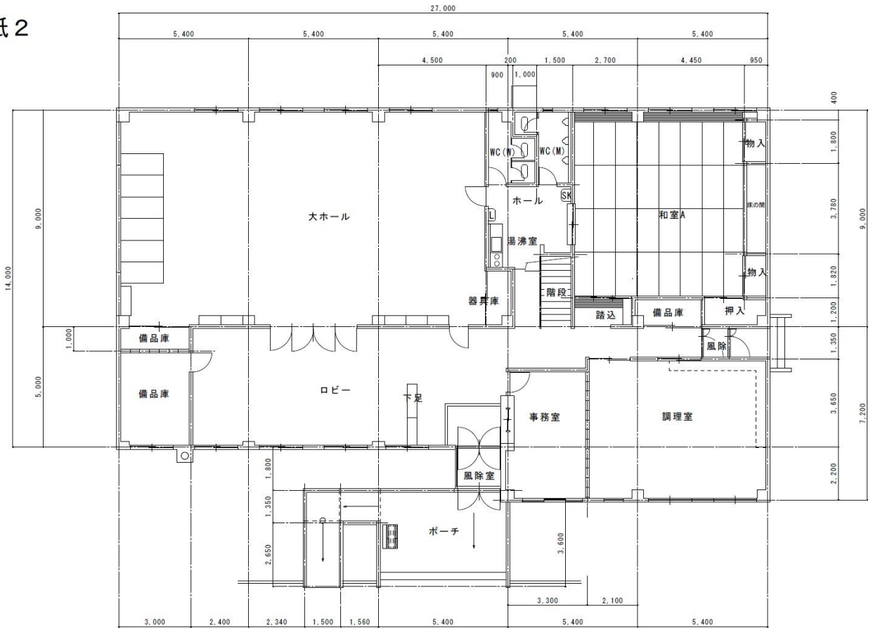
中央地区住民センター 1階平面図
