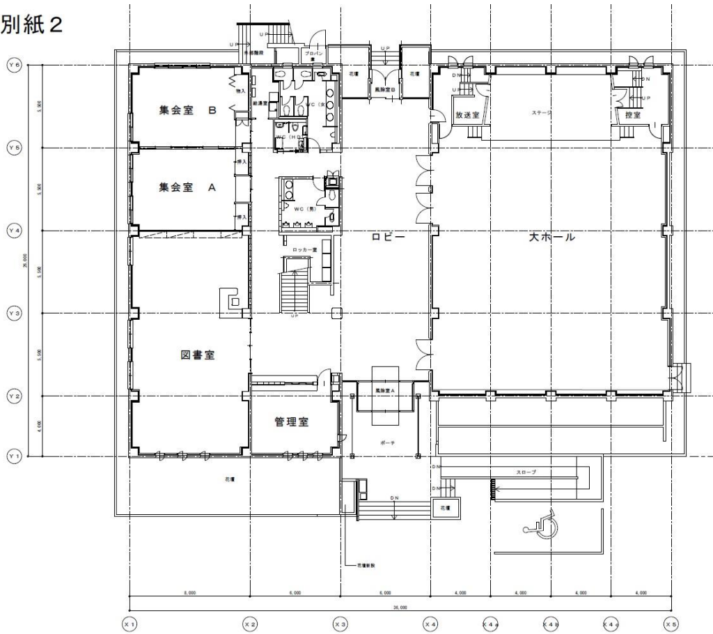
北野地区住民センター 1階平面図
