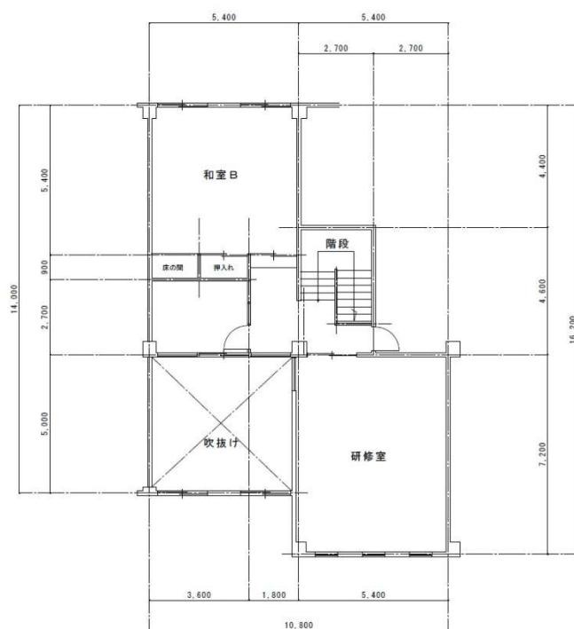
北成地区住民センター2階平面図
