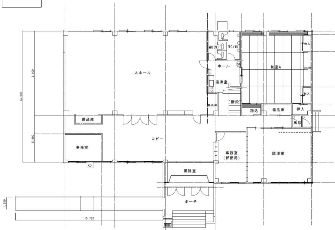
北成地区住民センター1階平面図
