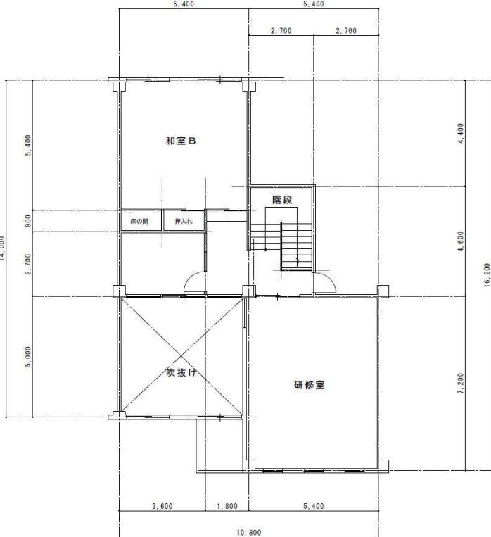
中央地区住民センター2階平面図
