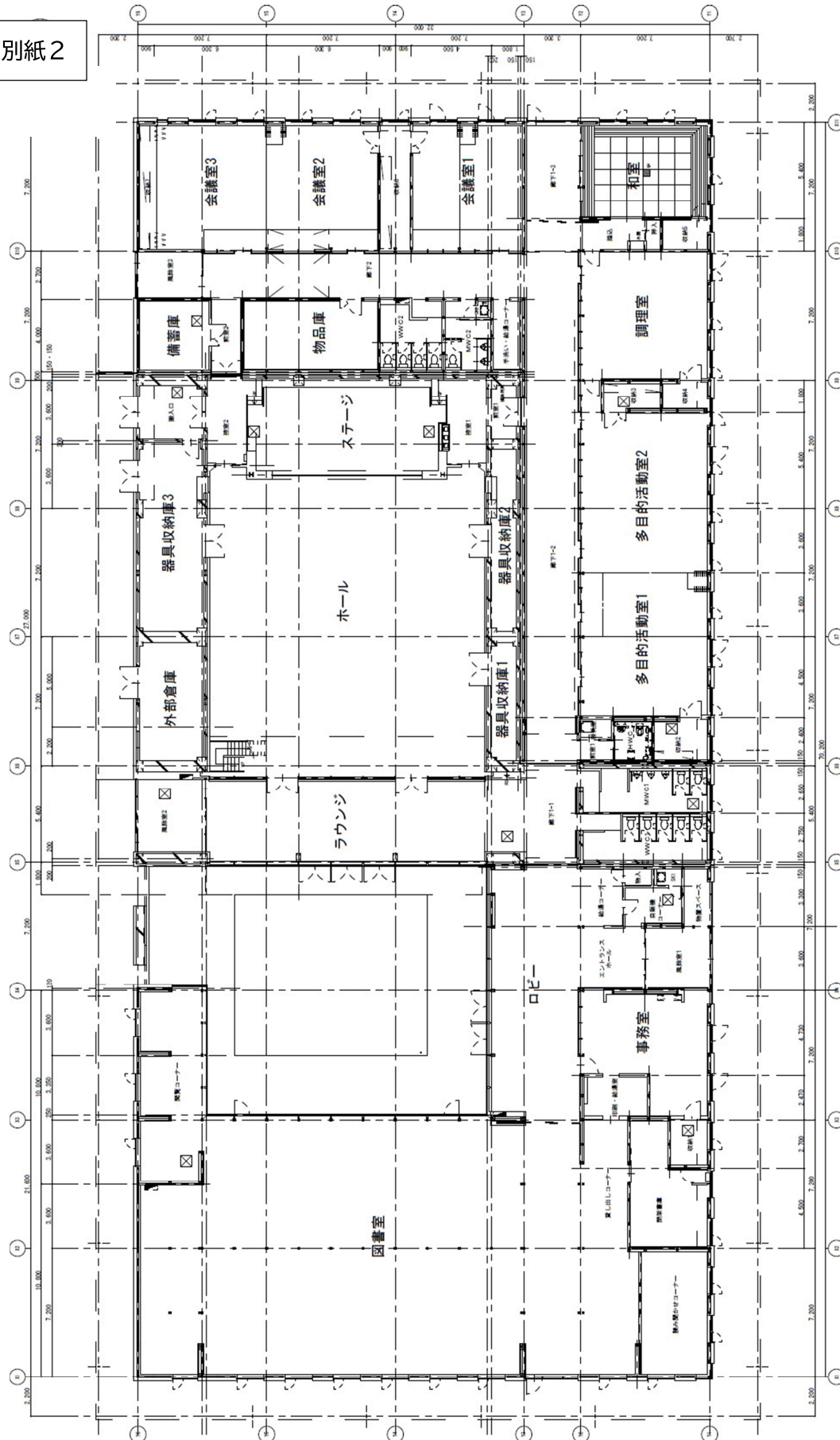
鷹栖地区住民センター平面図
